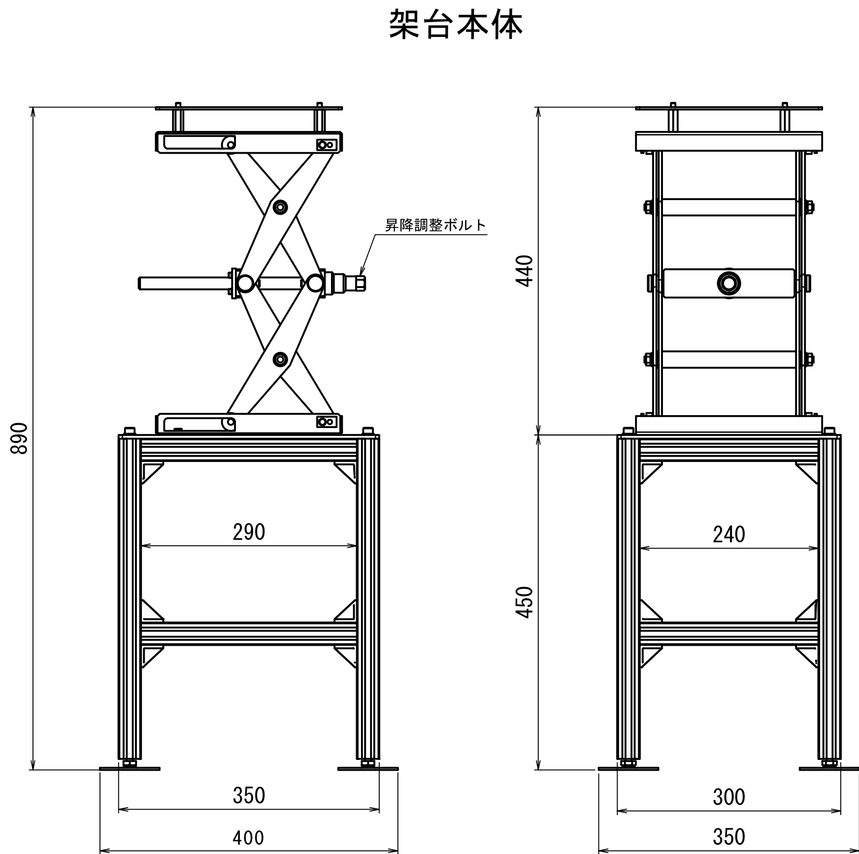
正面図
