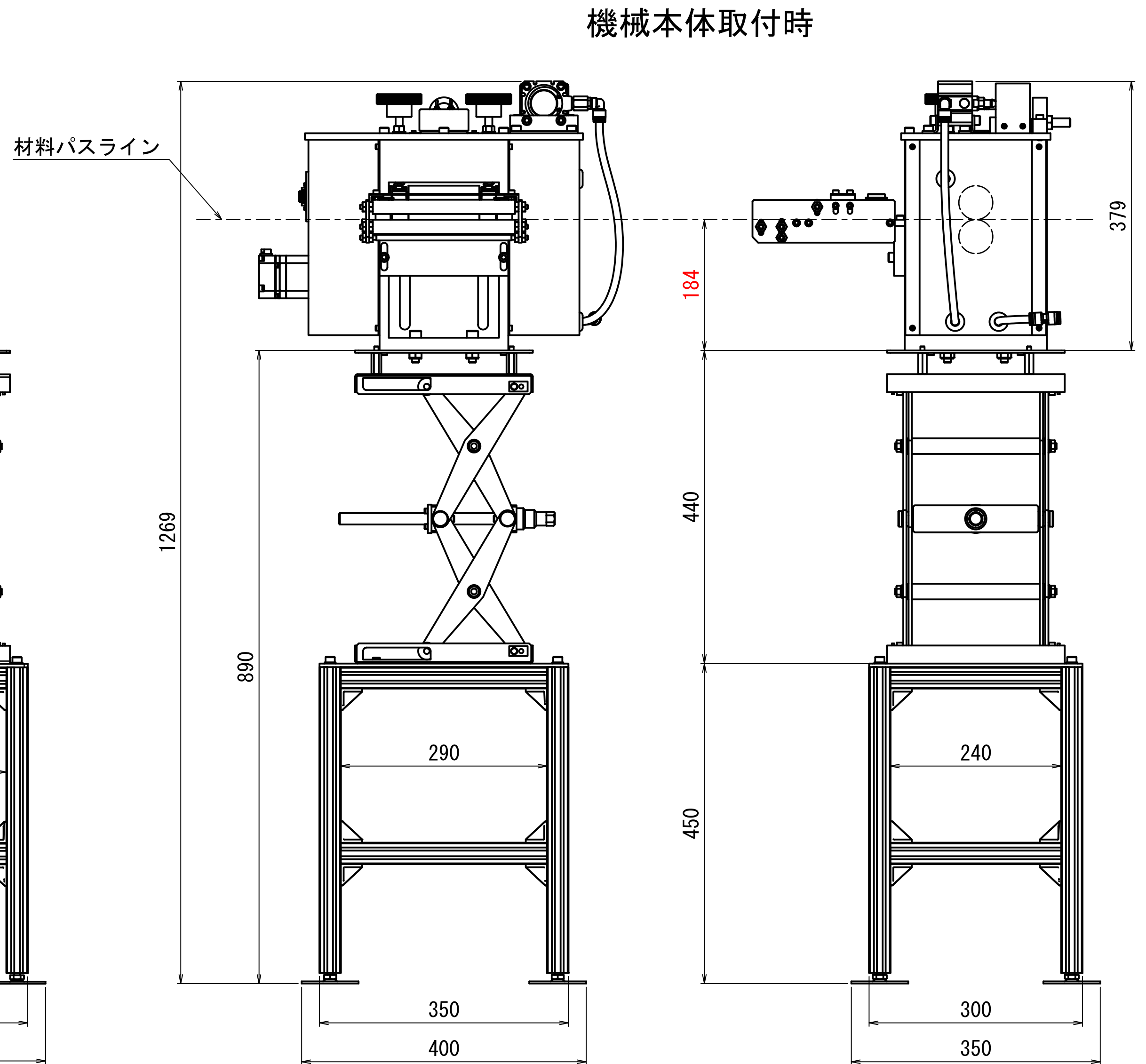
正面図
